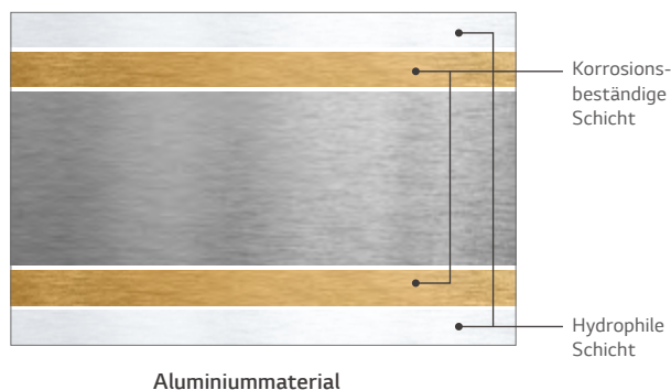
Aufbau der Lamellenwand
