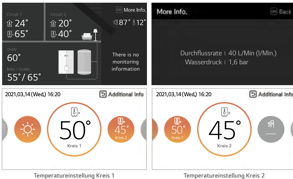
Temperatureinstellung Kreis 1
